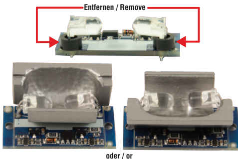
Abbildung 2: Einbau Reflektor
